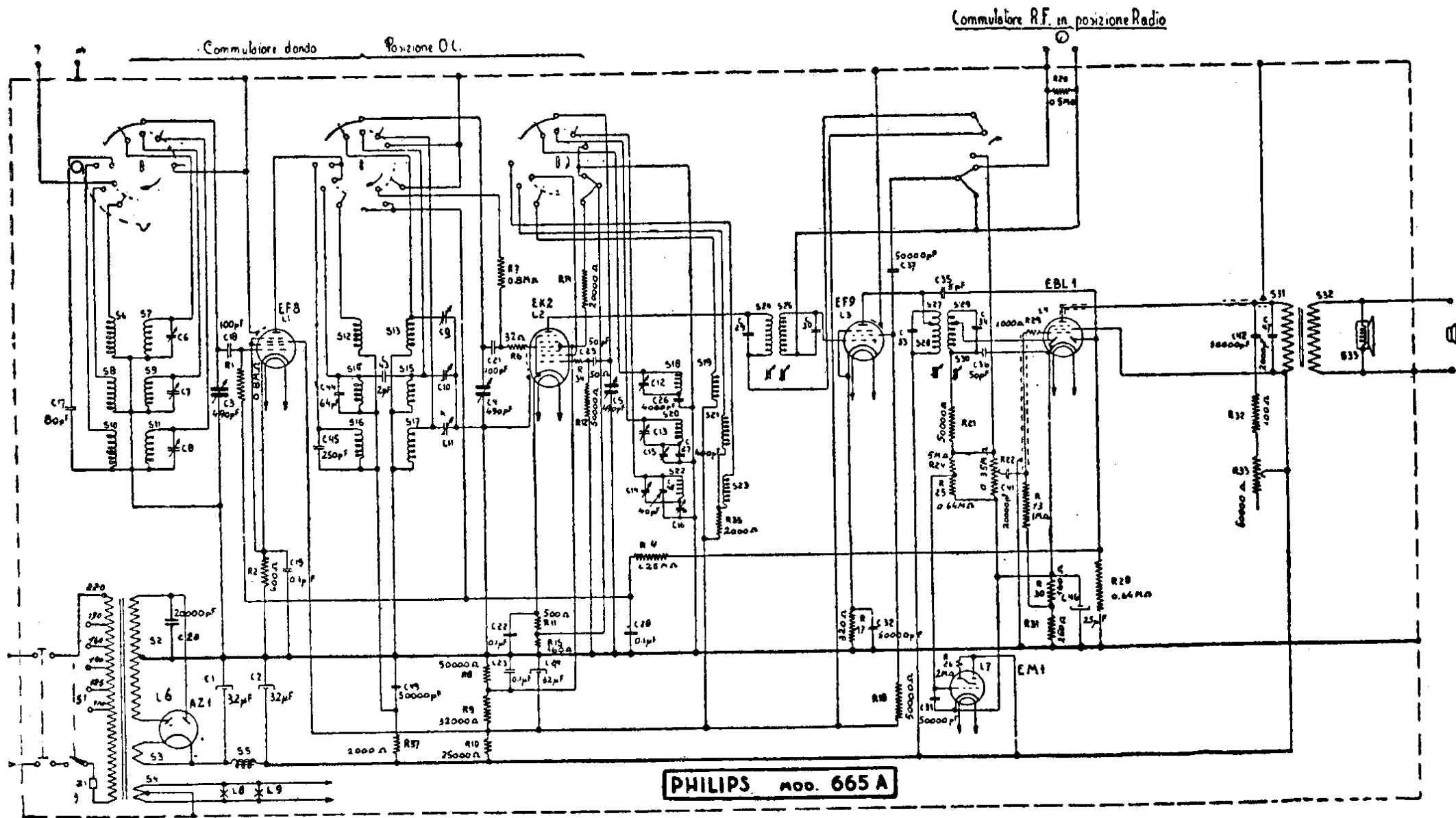
PHILIPS RADIO — Mod. 665 A — Produzione 1938-39. — Gamme: c. (18-51), m. (210-575), l. (200-2000). Media frequenza: 468 kHz.
